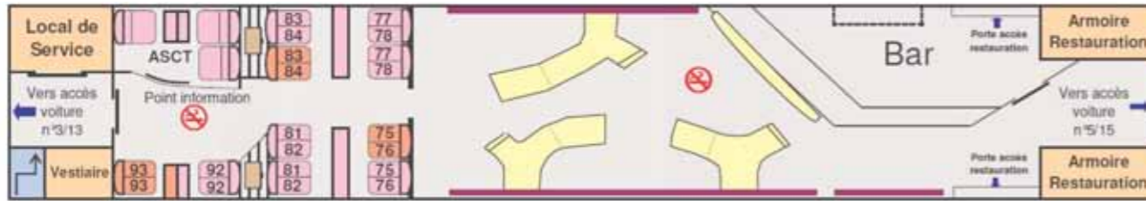
VOITURE N° 4 OU 14 - 2 ème classe, 10 places assises - BAR - Point information ASCT
